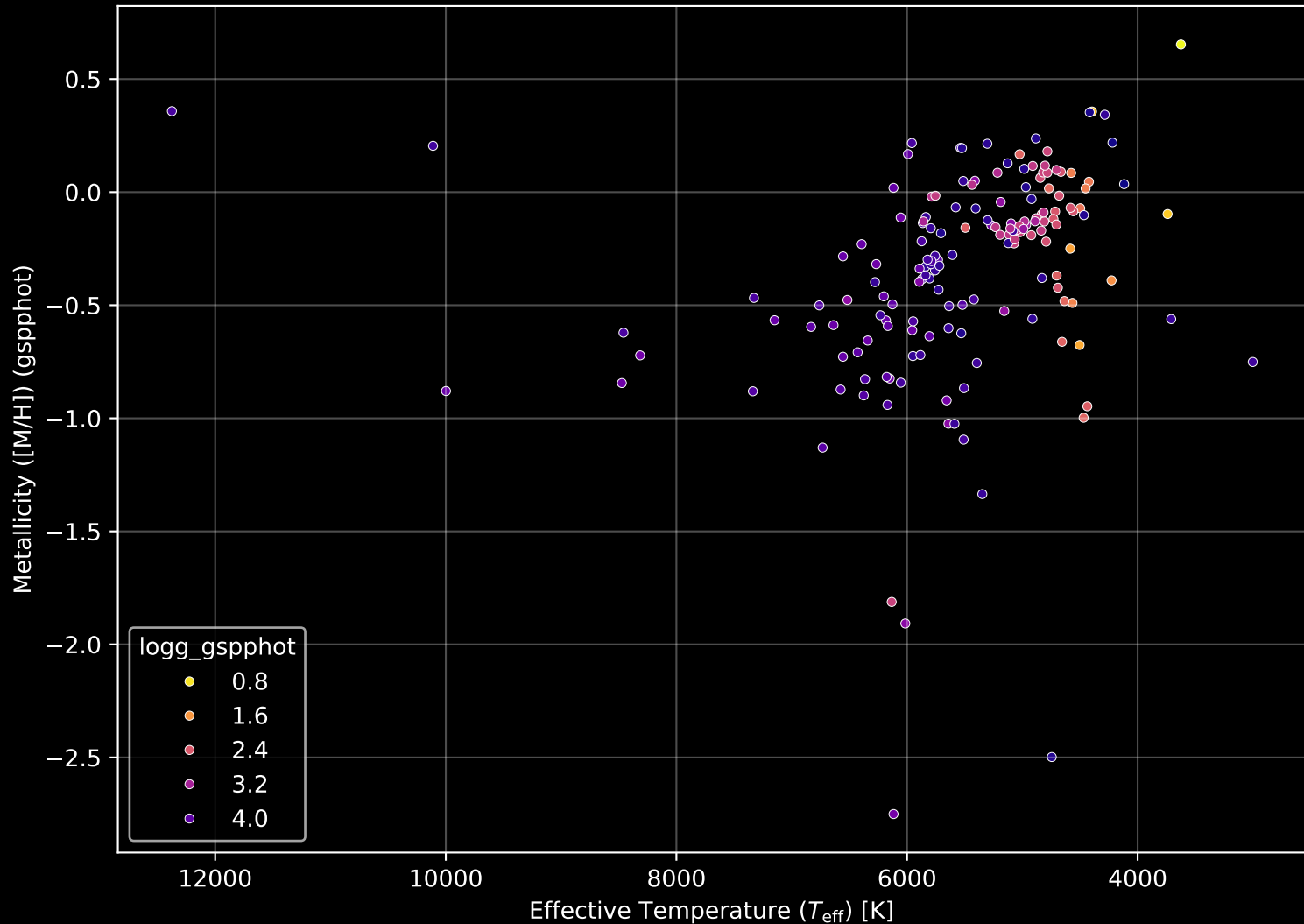
APOGEE DR17 Field: [275-19-O_TESS] Stellar Population Parameters (n= 166)
